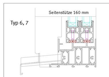
Schiebeanlage SH 2/2 HF, 2-läufig, 2-flügelig hinter Fixfeld, aus wärmedämmten Alu-Profilen
