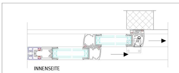
Schiebeanlage SH 2/2 HF, 2-läufig, 2-flügelig hinter Fixfeld, aus wärmedämmten Alu-Profilen
