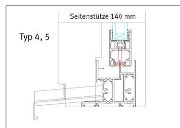
Schiebeanlage SH 2/1 HF, 2-läufig, 2-flügelig hinter Fixfeld, aus wärmedämmten Alu-Profilen
