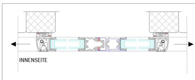
Schiebeanlage SH 2/1 HF, 2-läufig, 2-flügelig hinter Fixfeld, aus wärmedämmten Alu-Profilen
