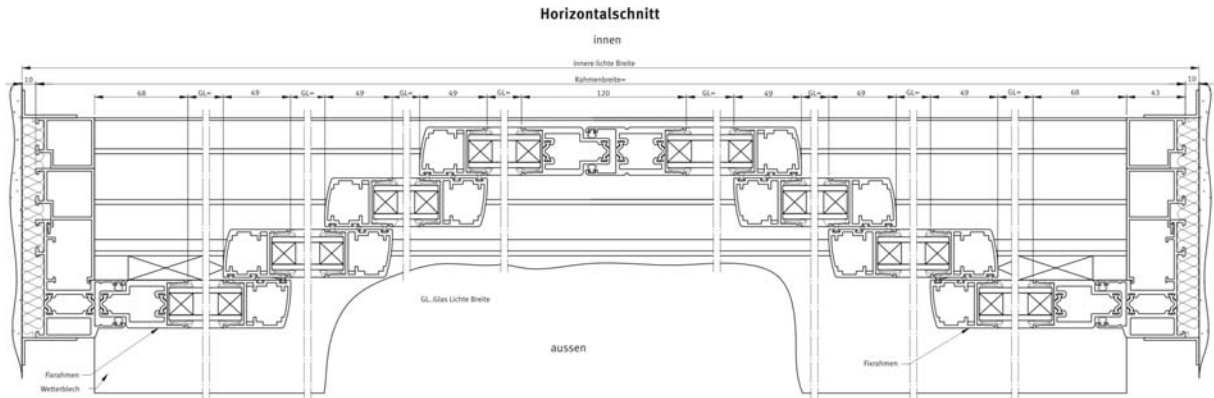
Schiebesystem SH 6/3 hinter Fixelement, wärmegeämmte Aluminiumprofile
